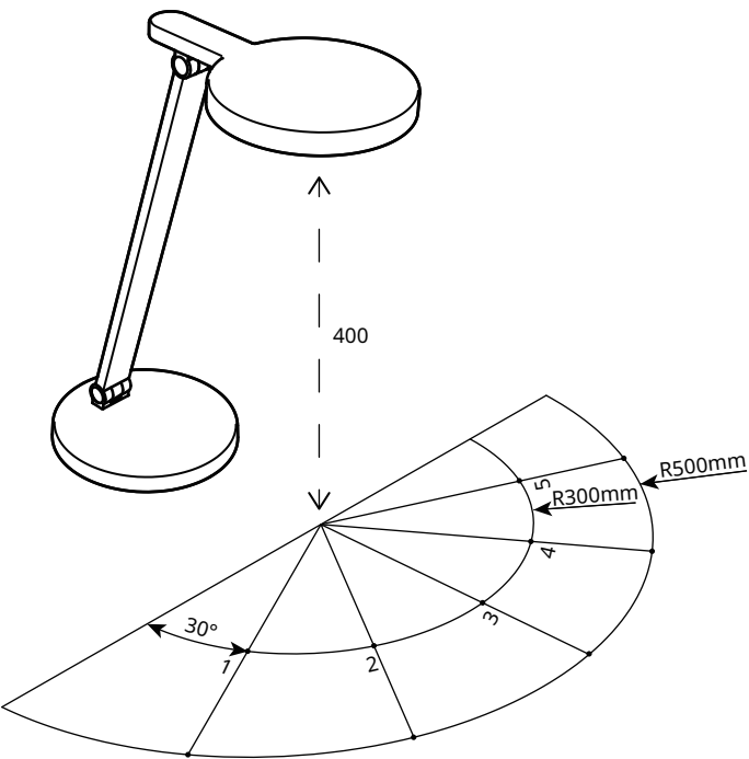
台灯处于正常工作位置，出光口面处于水平状态，出光口面与工作面垂直距离为400mm。
